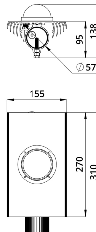
Габаритный чертеж
