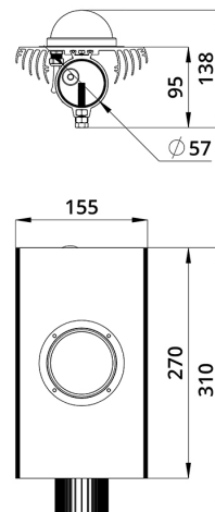
Габаритный чертеж
