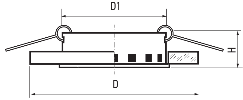
Рис. 1. Светильник PGX53d
